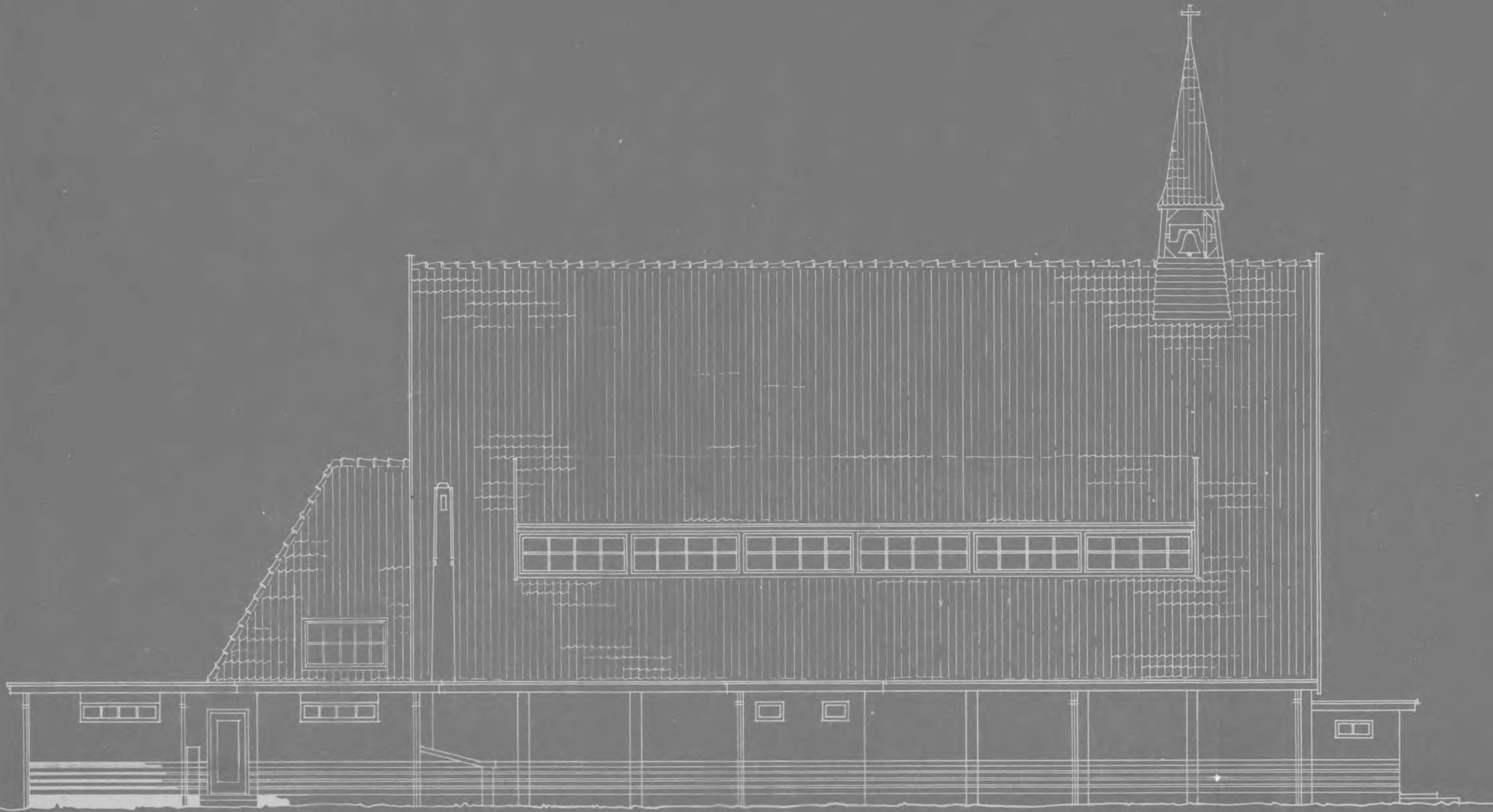
ZYGEVEL.
